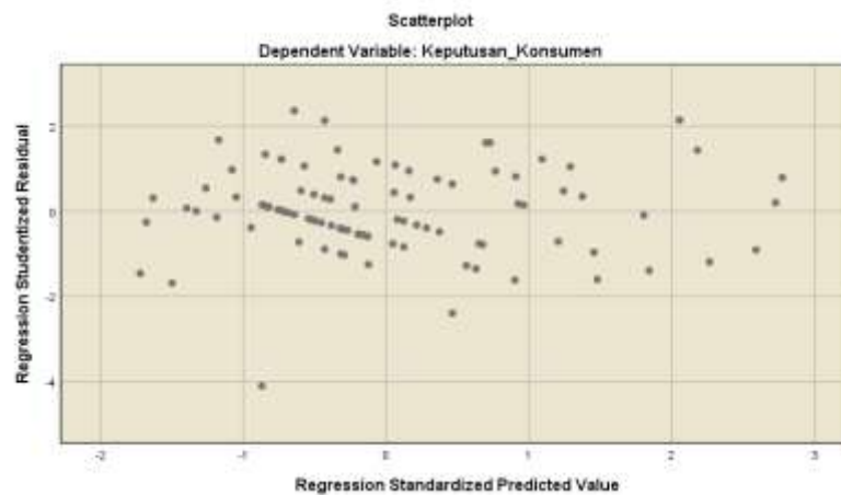
Gambar 3 Uji Heteroskedastisitas Sumber : Data diolah, 2021
